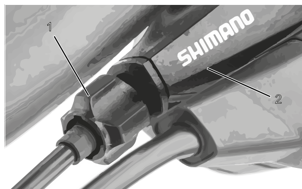
Figura 144: Boccola di regolazione (1) del cambio azionato da cavo singolo con scatola della leva del cambio (2), esempio
