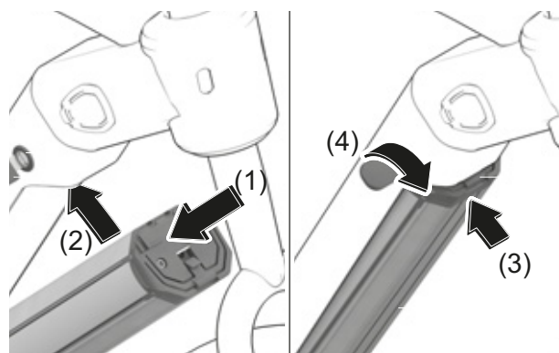
Figura 121: Montaggio della batteria integrata
