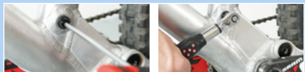
Figura 180: Fissaggio del perno Postpin
