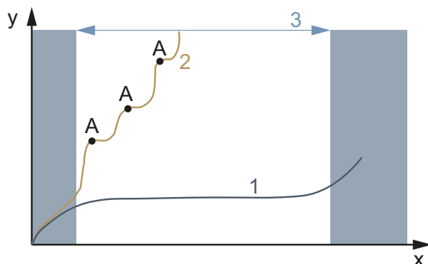
Figura 133: Diagramma dell'usura, asportazione di materiale (y) in funzione della durata di funzionamento (x)
