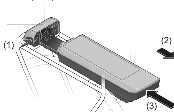
Figura 119: Smontaggio (2) e montaggio (3) della batteria sul portapacchi
