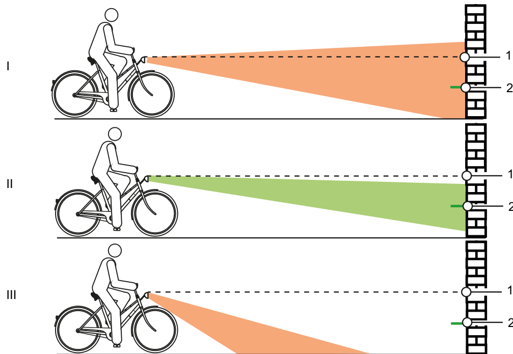
Figura 140: Luce regolata a un'altezza eccessiva (1), correttamente (2) e a un'altezza insufficiente (3)
