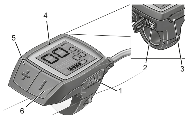
Figura 123: Struttura del computer di bordo BOSCH Purion
